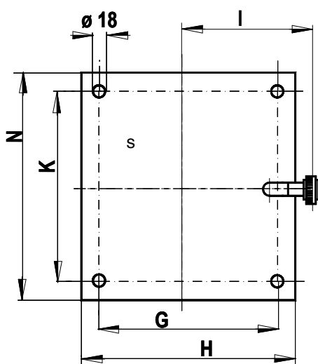
Размеры 32 - 50
