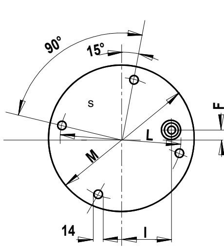
Размеры 15 -25
